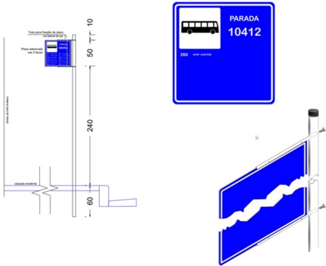
Exemplos Ilustrativos de Layouts
